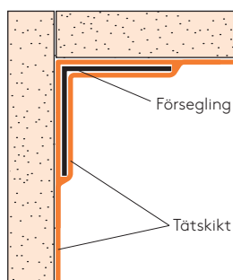
Figur 13. Hörn i skivvägg VTv.
