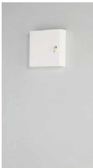
Medicinskåp med överfalsad, låsbar lucka samt en flyttbar glashylla B/H/D: 350/350/115 mm
